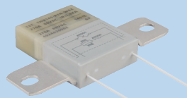
受控熔断器 (iTCO) 主动保护 过温度, 过电流
